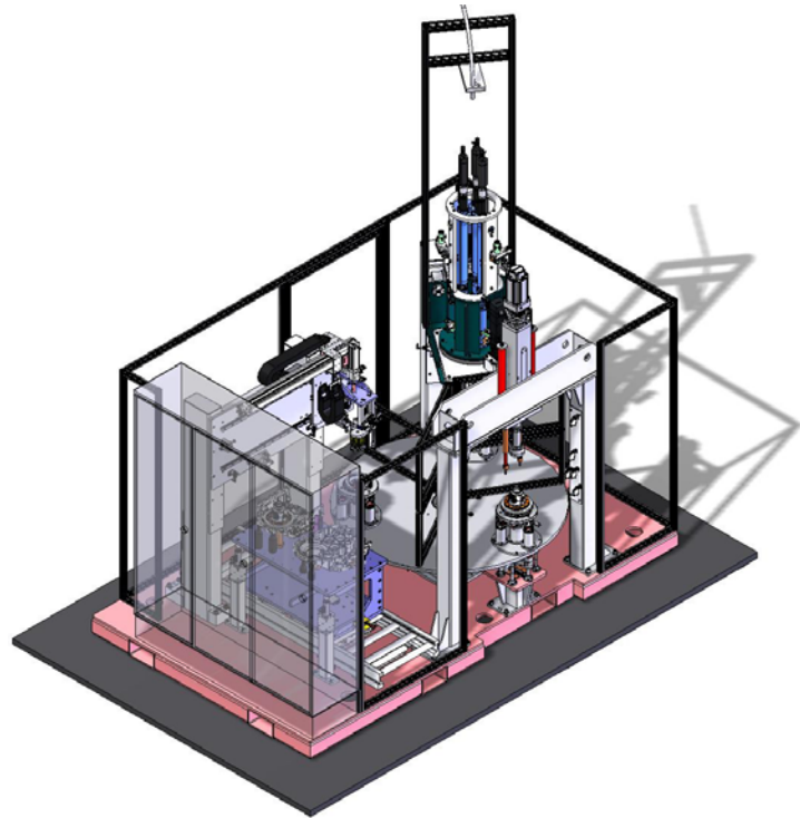
Getriebemontagestation
