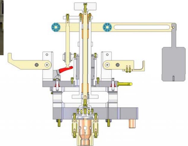
Schnittdarstellung der Axialspielmessvorrichtung
